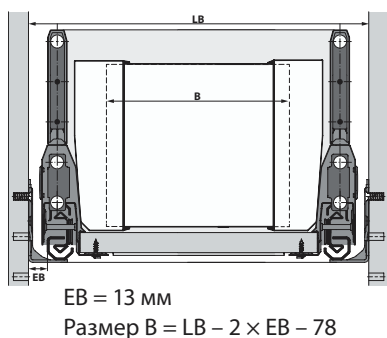
Размеры для раскроя для ArciTech
