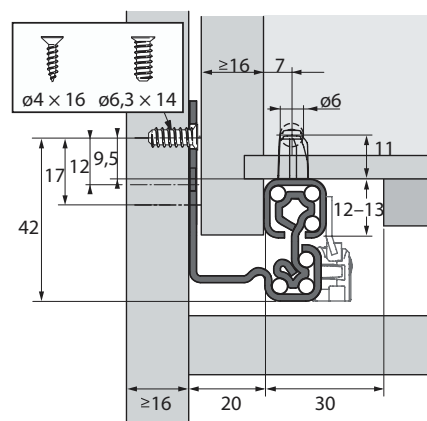
Размеры для монтажа Qudro V6+
