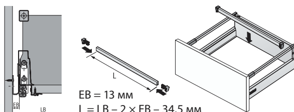
Монтажная схема
