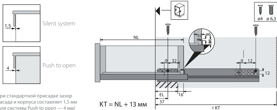
Размеры для монтажа
