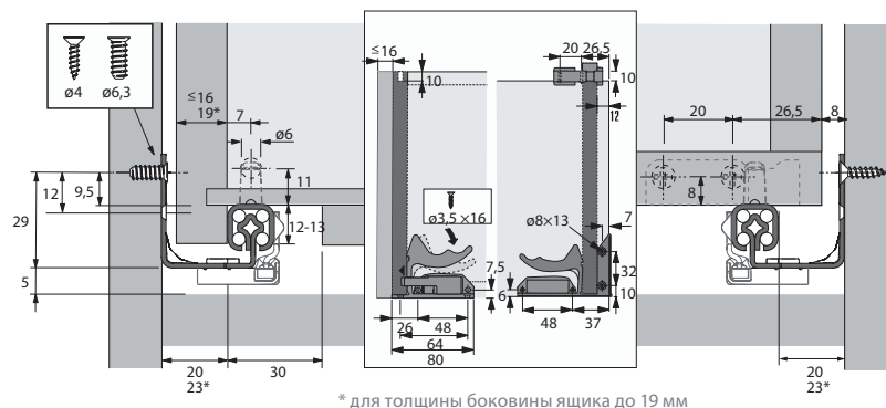
Размеры для монтажа
